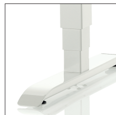
Mechanische Höhenschnellverstellung (L1) Verstellbereich: 720-1180 mm Hub: 460 mm
